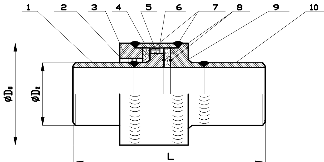
Rys. 1 Złącze izolujące t. ZIS (bez iskrownika)
