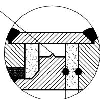
Iskrownik toroidalny
